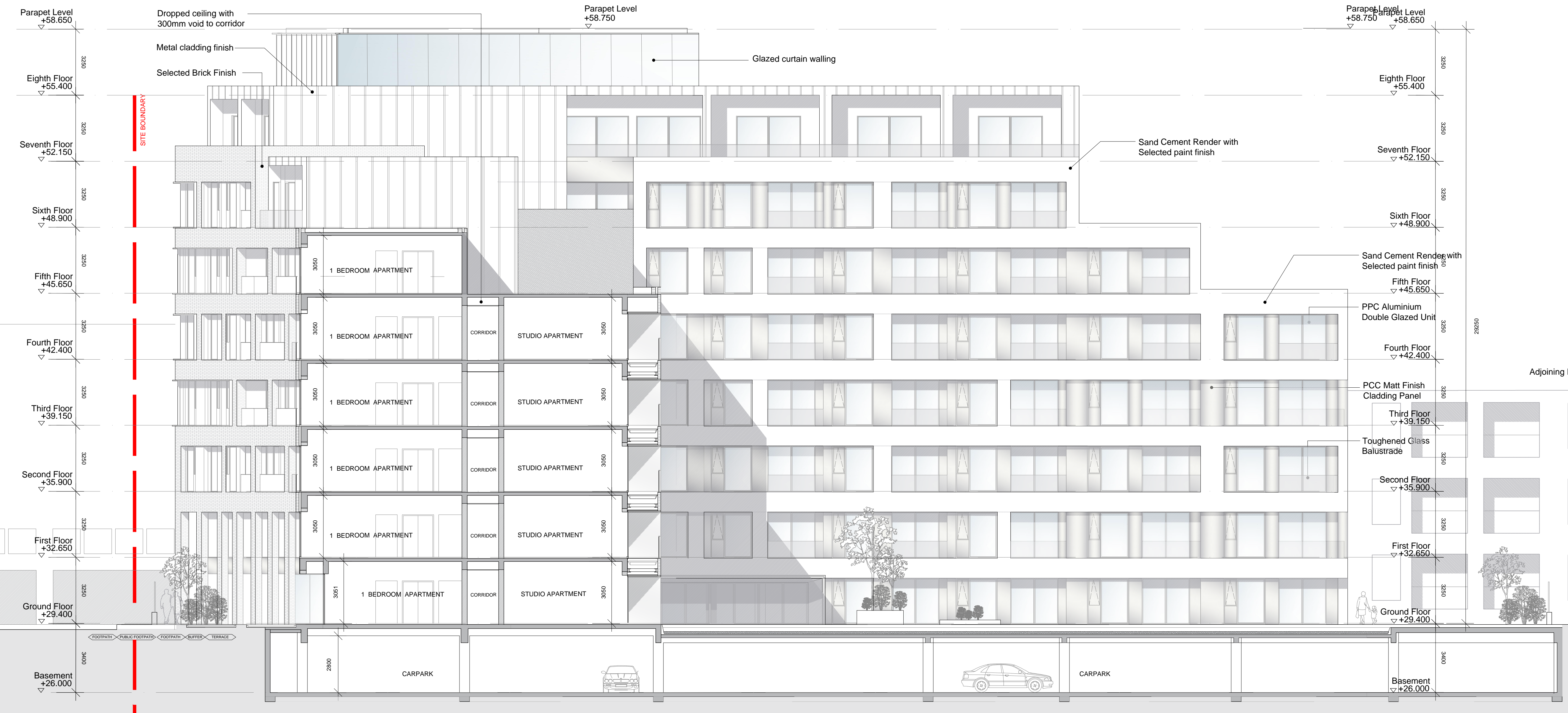
SECTION A-A - Scale 1:100@A1
